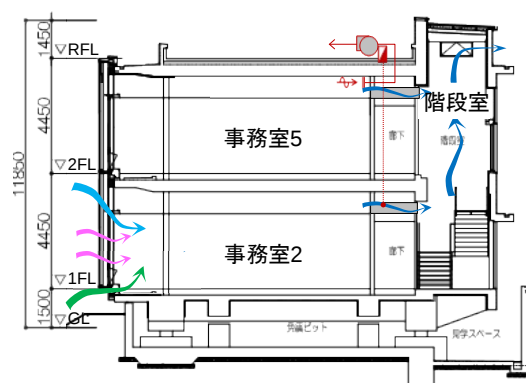
図-1 自然換気システム概要 (断面)
