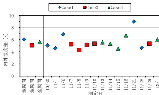
図-6 内外温度差の全期間および日平均
