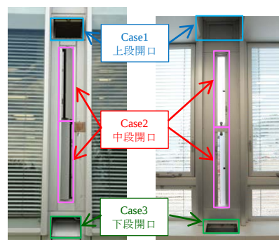
写真-1 自然換気パネル (左: 屋外側, 右: 室内側)
