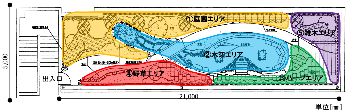
図-1 屋上ビオトープの平面図
