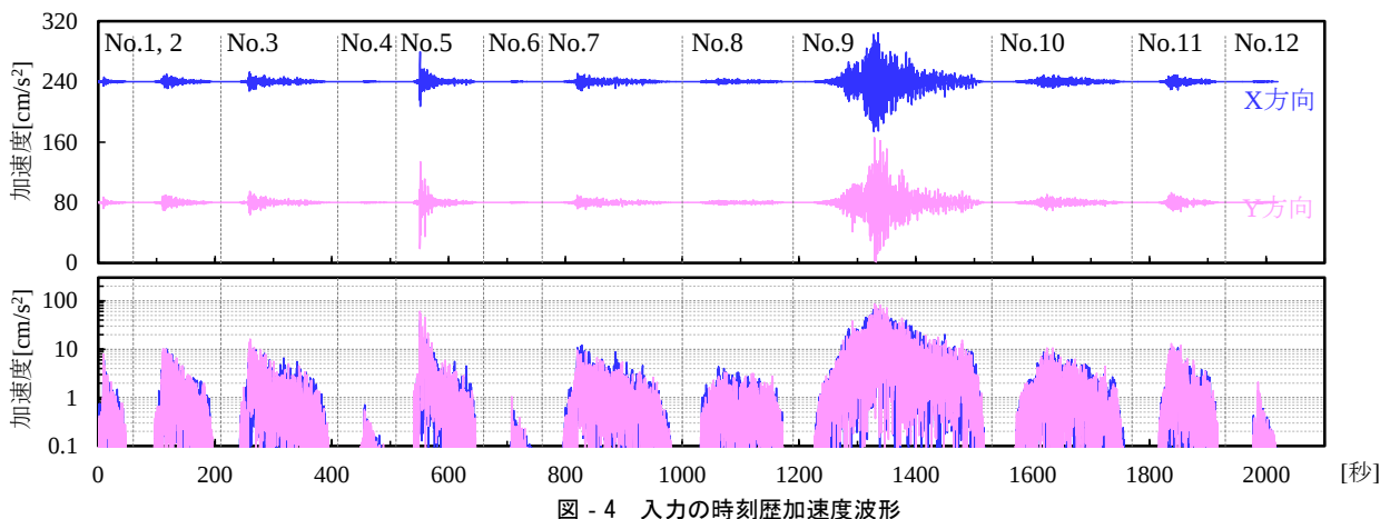
図 - 4 入力の時刻歴加速度波形
