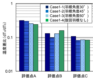
図-6 温度差比
