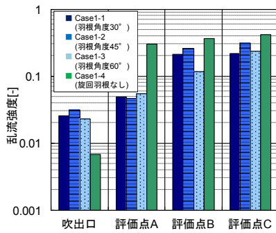
図-9 乱流強度
