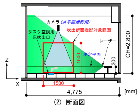
図-4 可視化実験概要図
