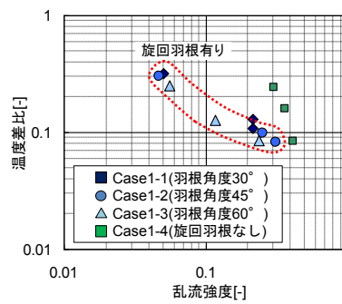
図-10 乱流強度と温度差比の関係
