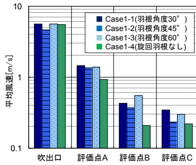
図-7 平均風速
