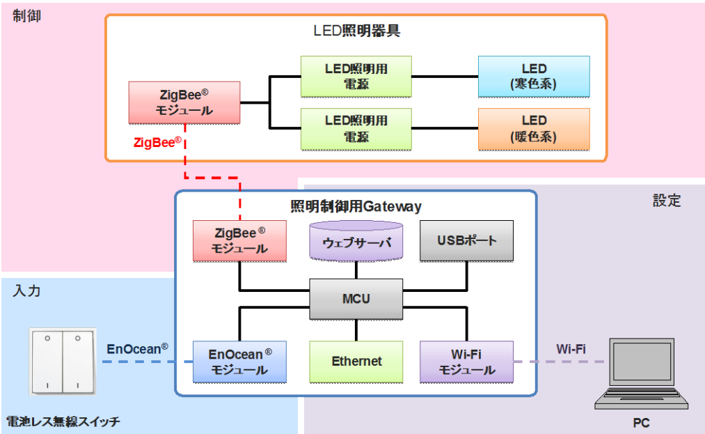
図ー1 照明システムの概念
