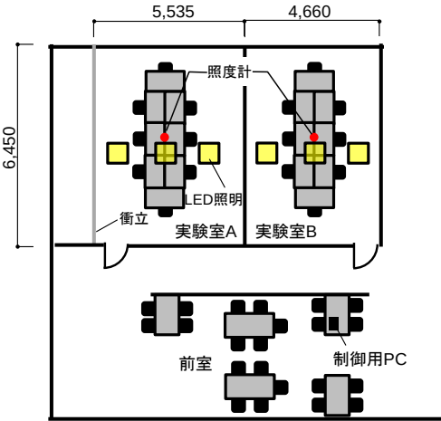
図-2 実験室平面図
