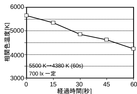
図-5 設定変更時の照明色温度
