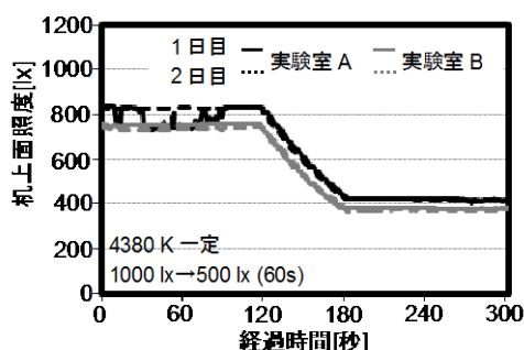
図-4 設定変更時の机上上面照度
