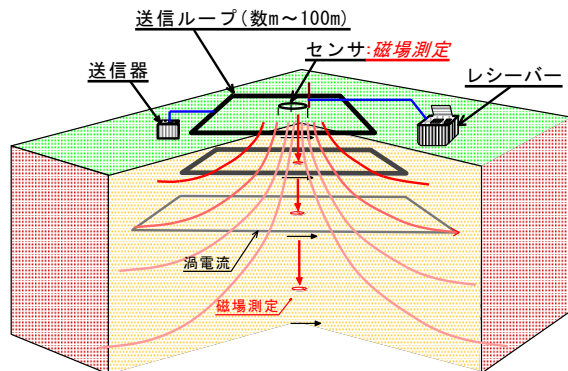
図 TDEM 法の探査原理
